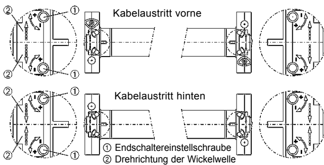
Abb. 4 Detailansicht Endschaltereinstellung
