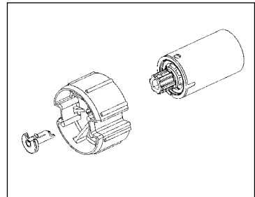
Afbeelding 2: Koppelingsbeveiliging*
