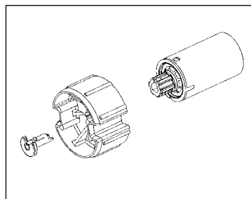
Figure 2: verrouillage de sécurité de l'accouplement*
