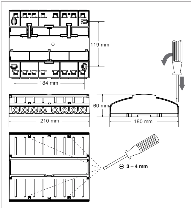
Abb. 4 Abmessungen AP-Gehäuse
