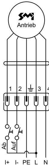
Tasterbetrieb (Einstellvorgang)
