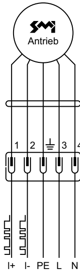
Telegrammbetrieb (Betrieb am Aktor)
