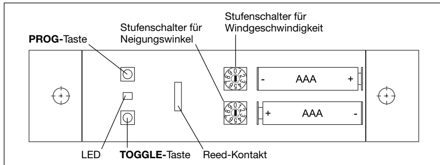
Bild 1: Gehäusehaube – Ansicht innen auf die Platine
