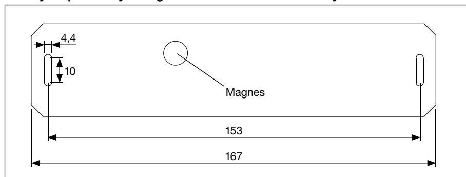
Rys. 2: Płyta podstawy – wymiary otworów montażowych
