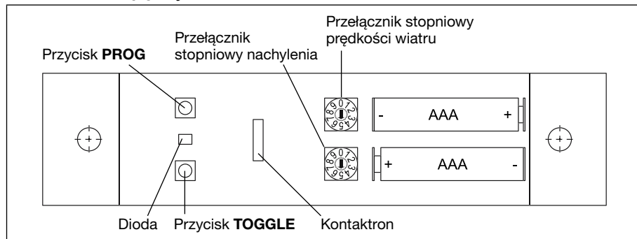
Rys. 1: Obudowa – widok wnętrza z płytą
